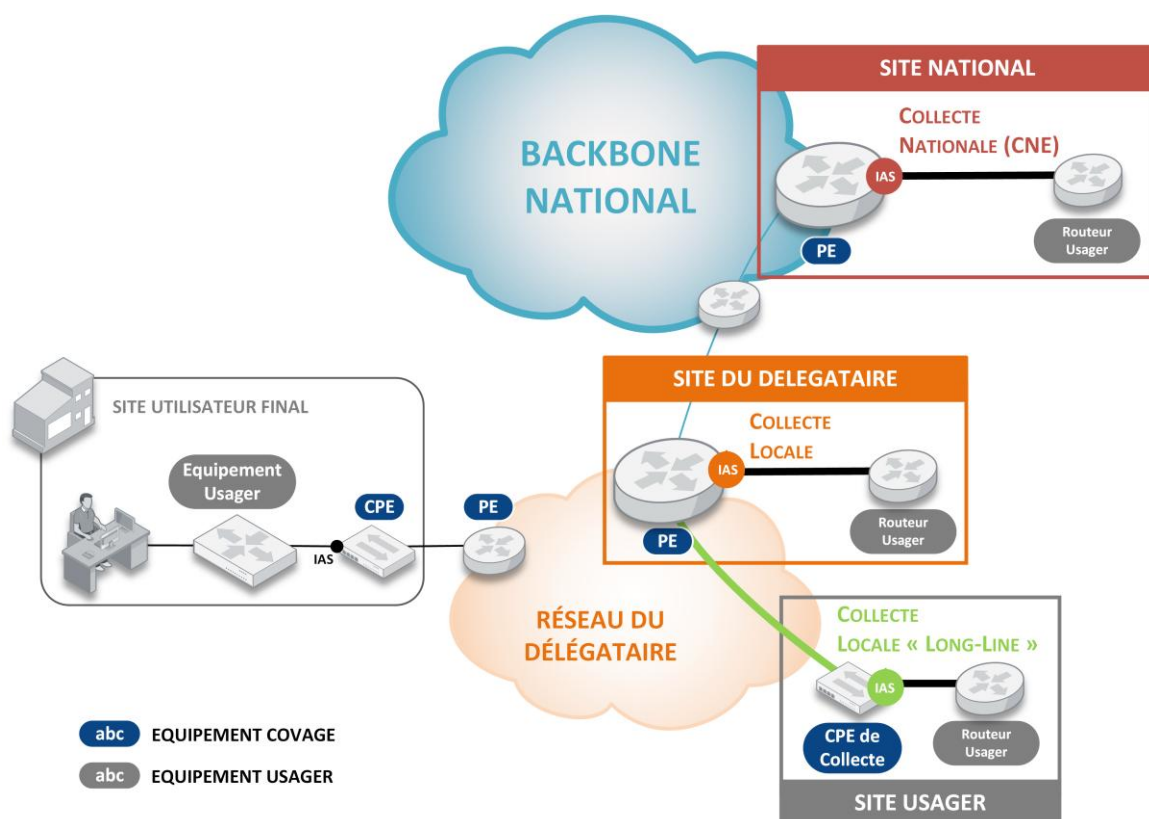
Figure 2 - Collecte Nationale / Locale
